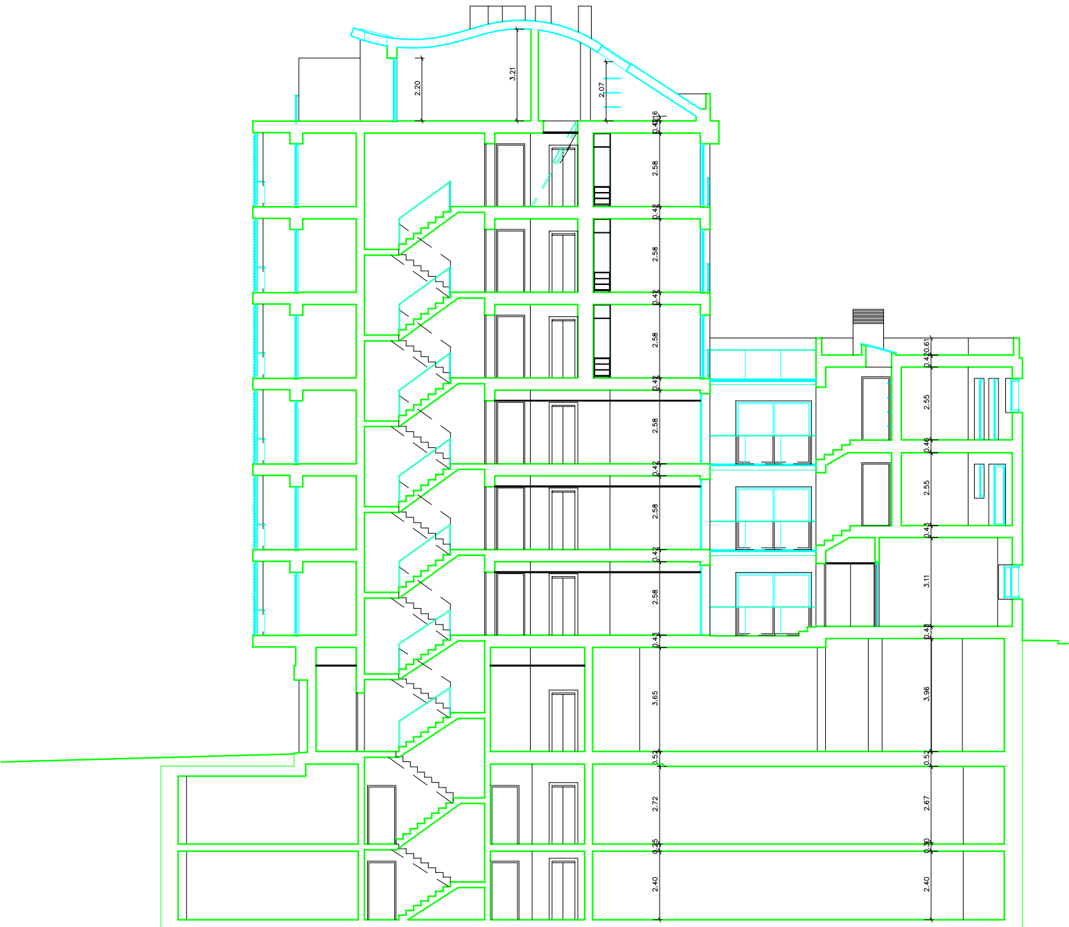
CORTE LONGITUDINAL
