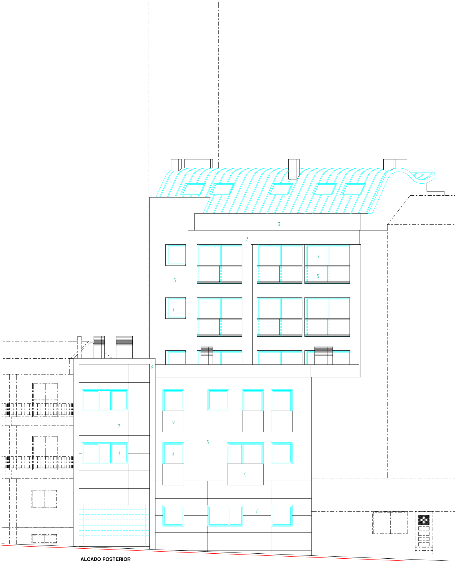
ALÇADO POSTERIOR
